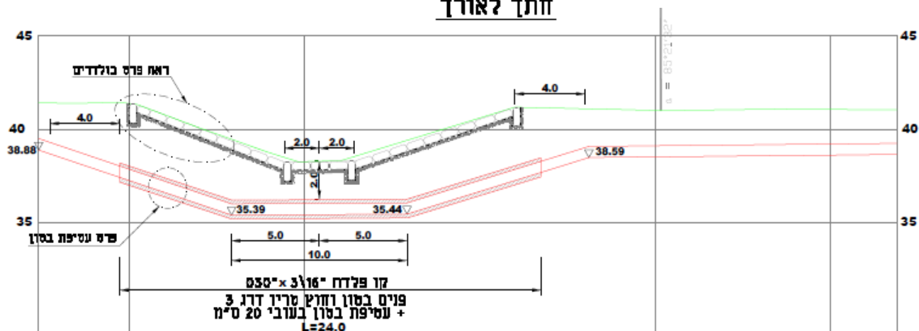
חתך לאורך
