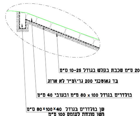
פרט בולדריים
