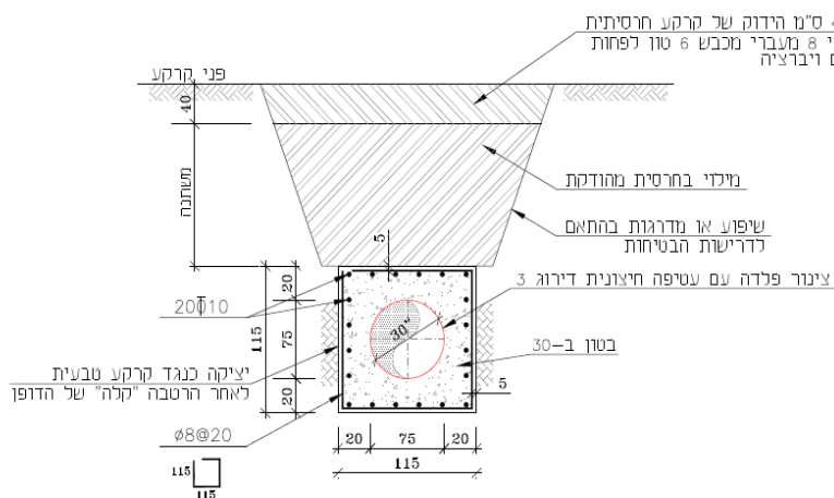
חתך טיפוסי לעטיפת בטון
